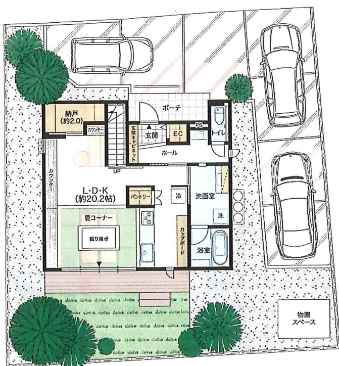
■1F平面図
