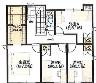
■2F平面図
